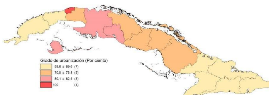
Mapa 3. Grado de urbanización por provincias. Año 2023
